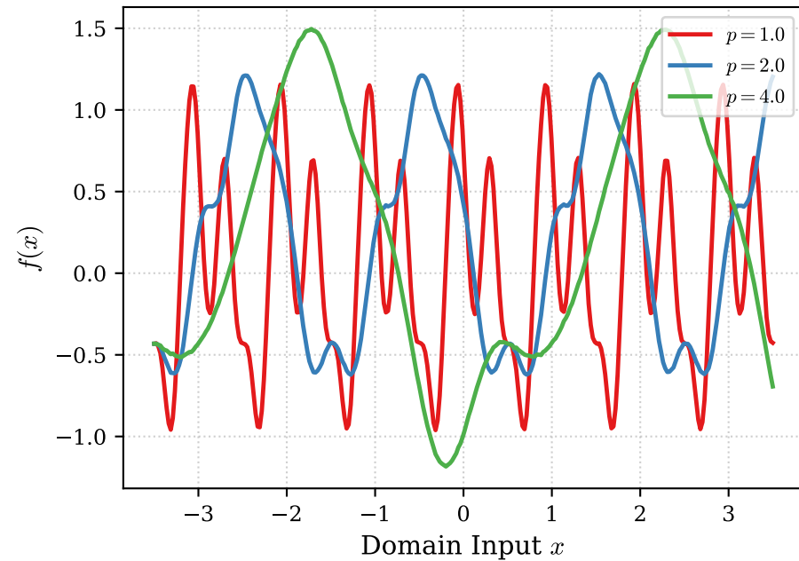
(d) Periodic: Variasi Periode p
