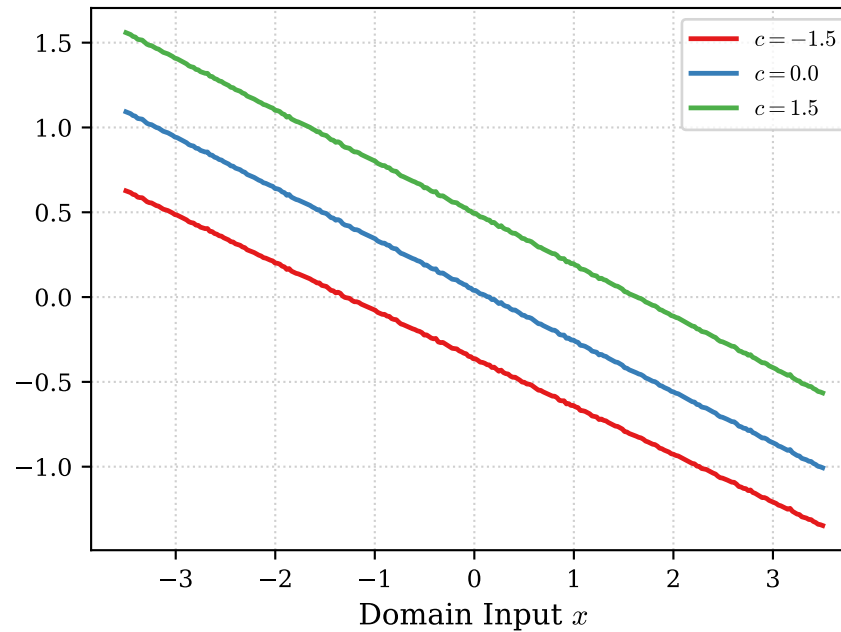
(e) Linear: Variasi Titik Tumpu c
